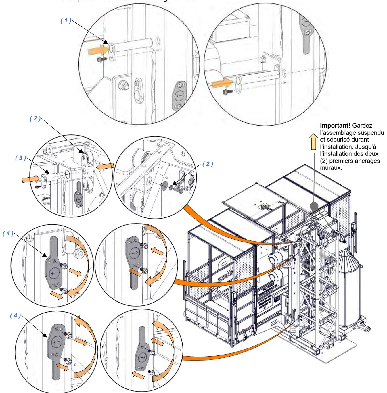
Figure 14 – Fermeture du garde-tour
