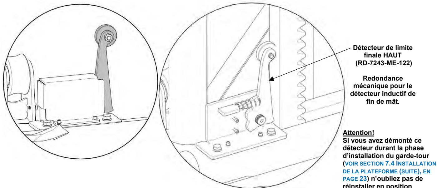
Figure 30 - Détecteur de limite finale HAUT
