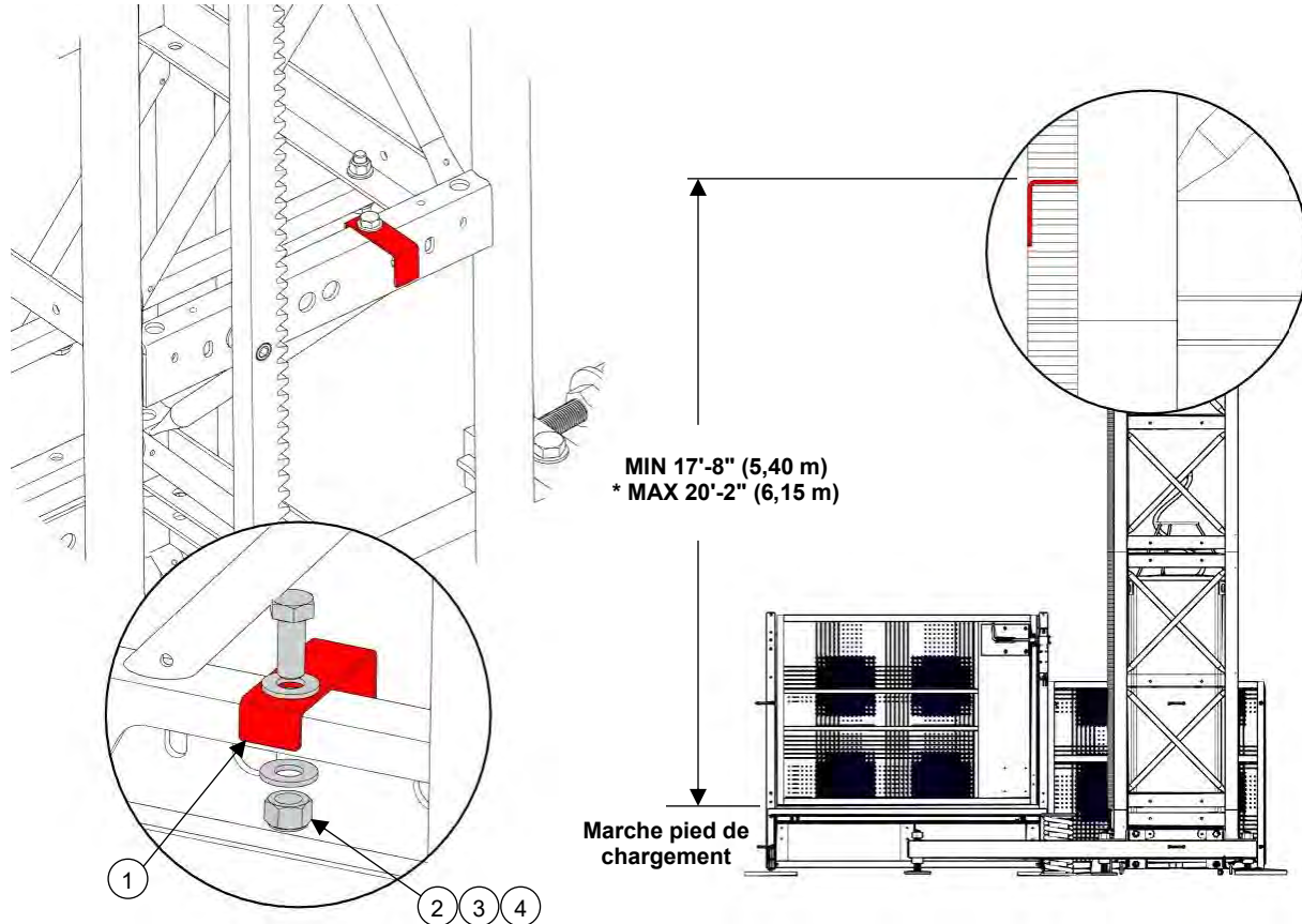
Figure 27 - Installation du patin du détecteur 10'-0" (3,0 m)
