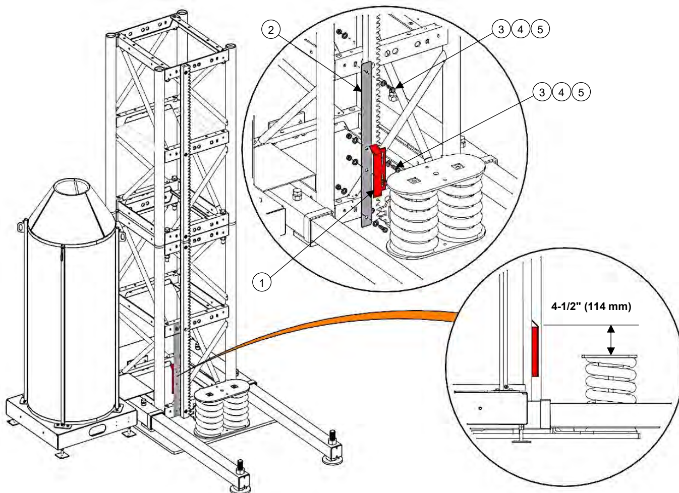
Figure 26 - Détecteur des amortisseurs
