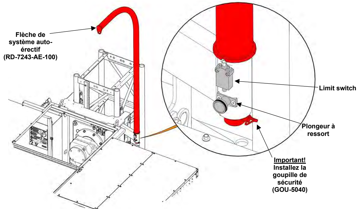
Figure 23 - Installation du système auto-érectif
