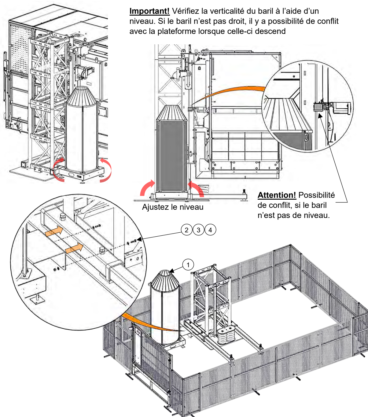
Figure 6 - Installation du baril pour câble
