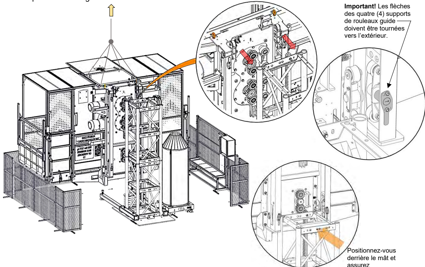
Figure 13 - Installation de la plateforme sur les premières sections de mât
