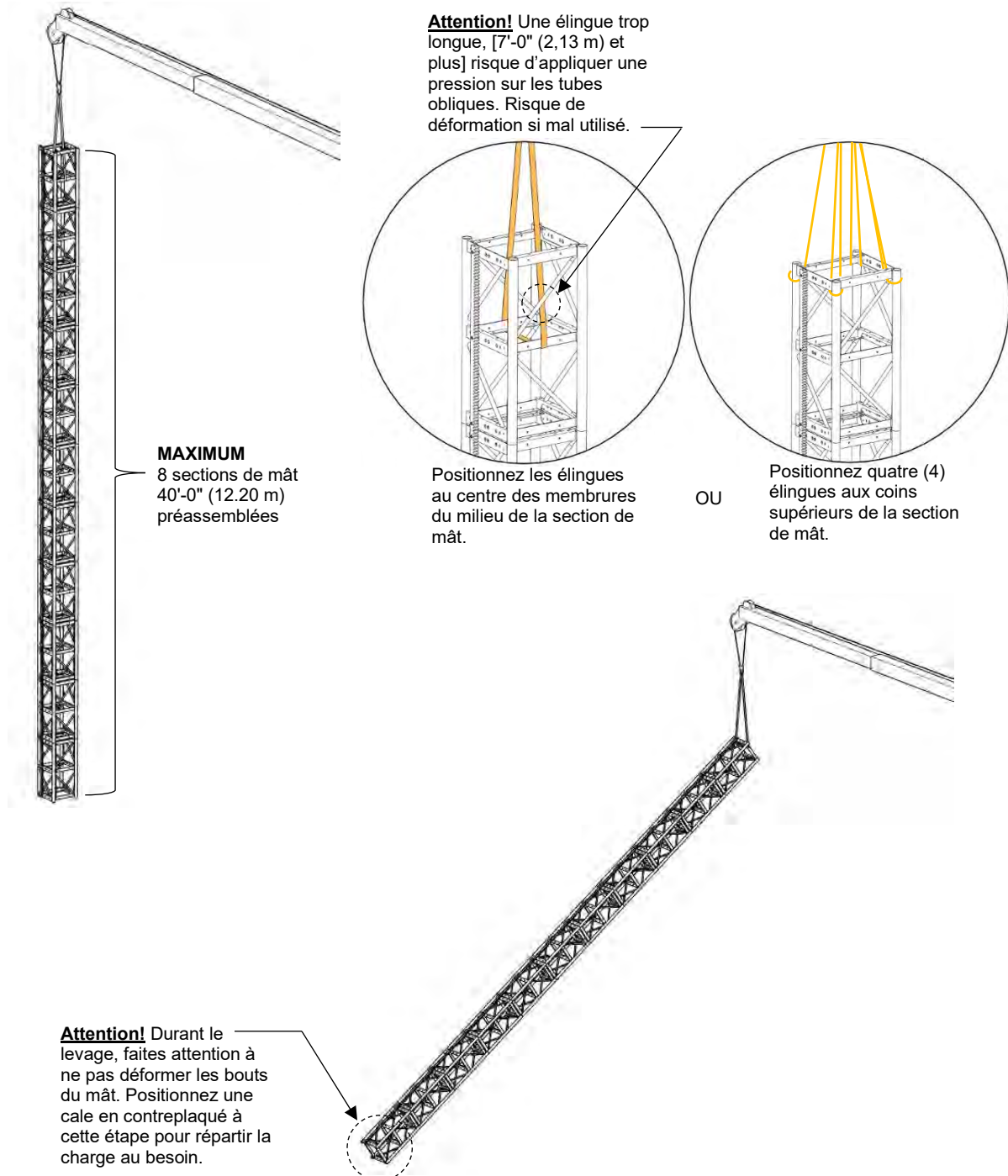
Figure 15 - Élingage des sections de mât
