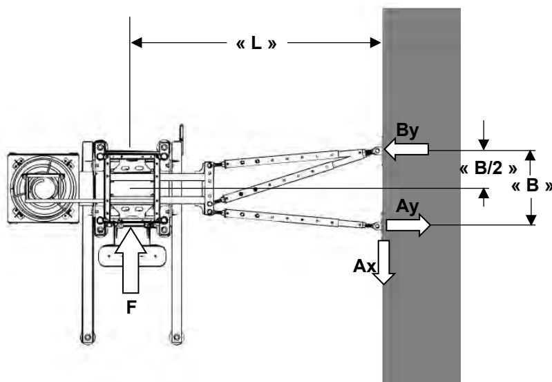
Figure 21 - Dimensions et efforts au mur
