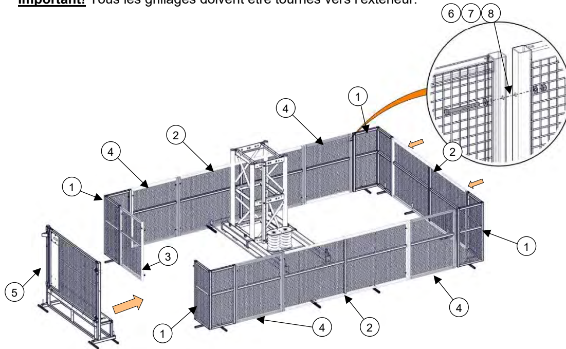
Figure 4 - Installation du grillage au sol
